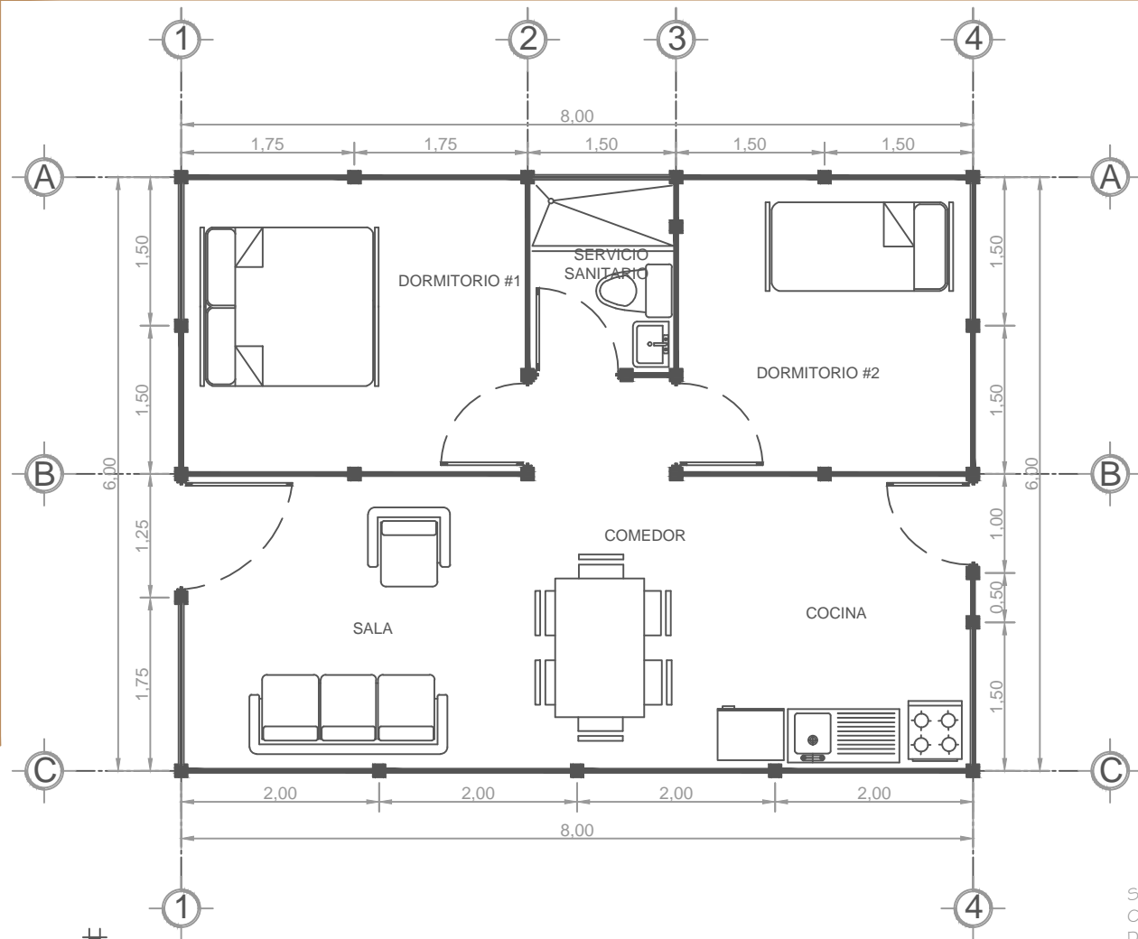
VIVIENDA TIPO I-D
